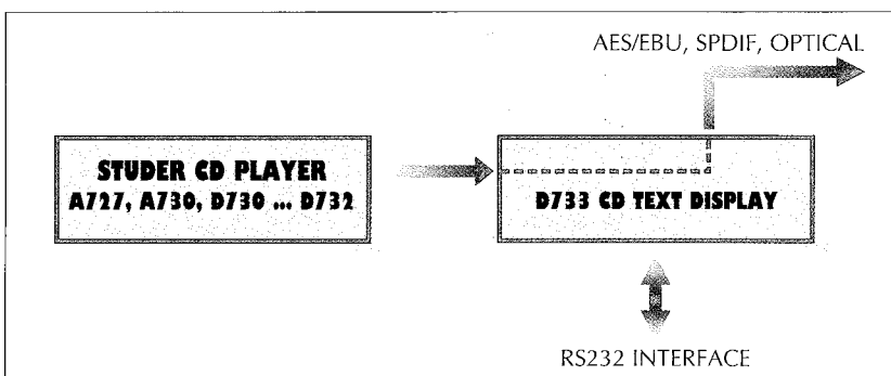
Blockschaltbild
