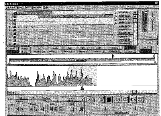
Abb. 5: Editor-Bildschirm
